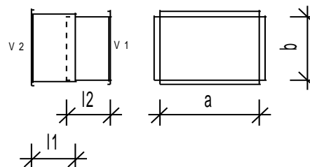
Schiebstutzen
